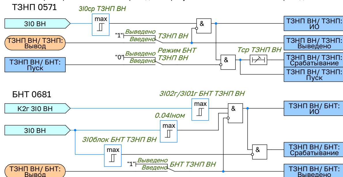
Рисунок 2.1 – Функциональная схема логики ТЗНП ВН
