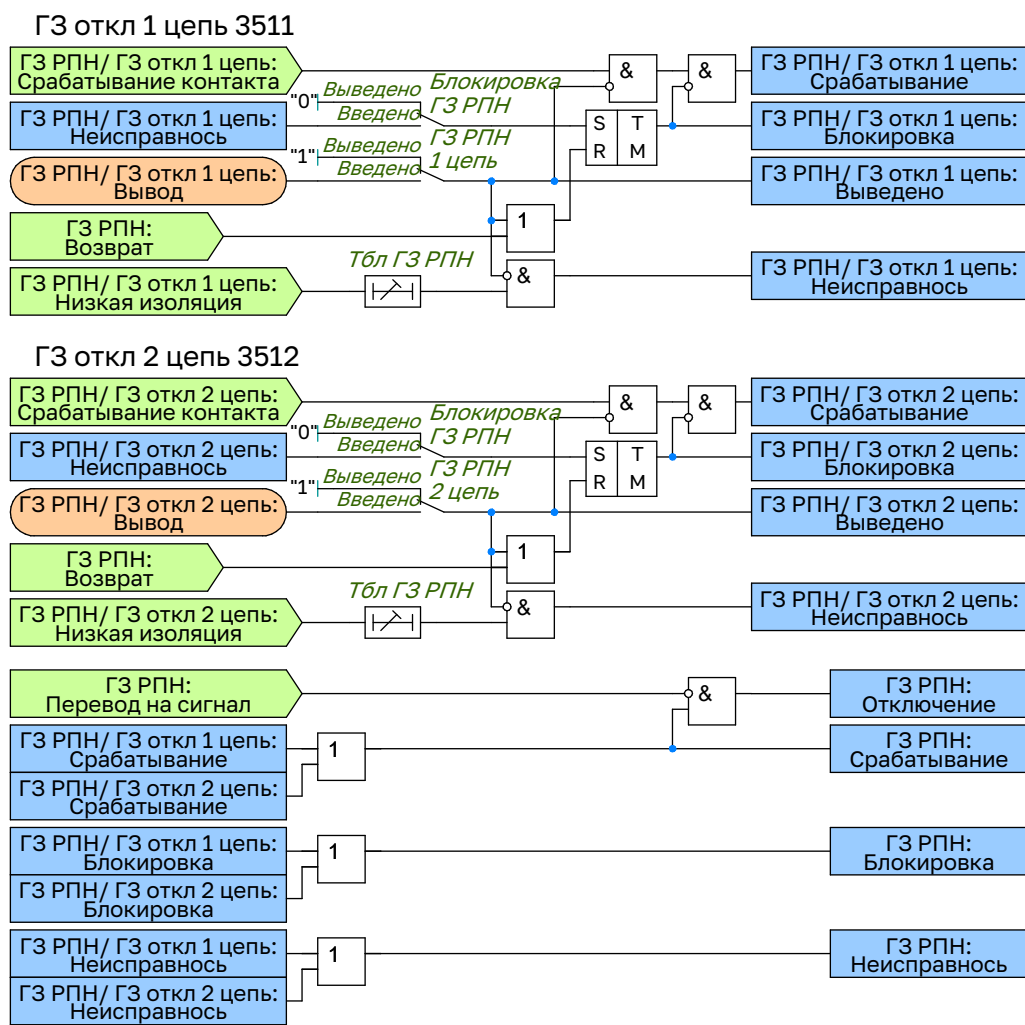
Рисунок 2.16 – Функциональная схема ГЗ РПН
