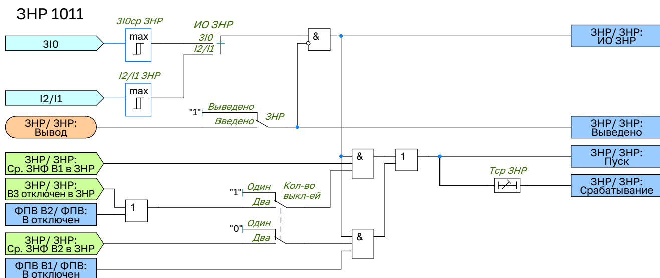
Рисунок 2.9 – Функциональная схема логики ЗНР
